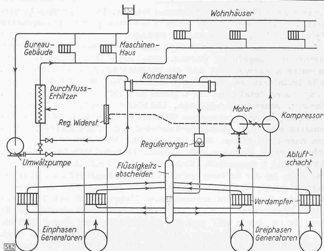
Schema der Abflus-Wärmepumpenanlage Altendorf des Etzelwerkes
