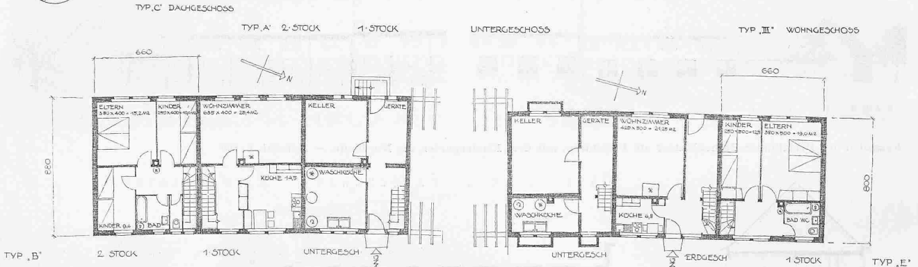
Vierzimmer-Einfamilienhäuser der Längsreihe 5.
