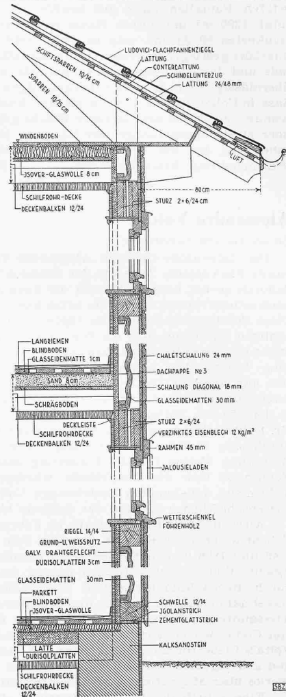
Abb. 5. Konstruktions-Einzelheiten 1:30
