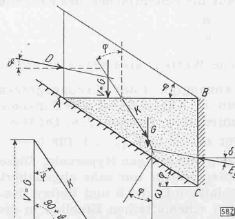
Abb. 8. Spezialfall der Gleitdruckberechnung: Felsneigung \omega = Böschungswinkel \varphi
