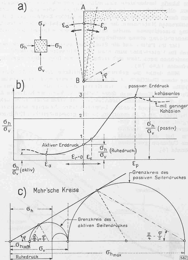
Abb. 4. Abhängigkeit des spezifischen Erddruckes von der relativen Bewegung zwischen Stützwand und Erdkörper (Schema)
