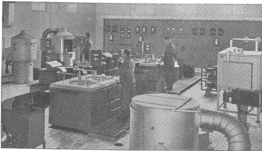
Meß- und Regeltafel in einer Werkzeughärterei
