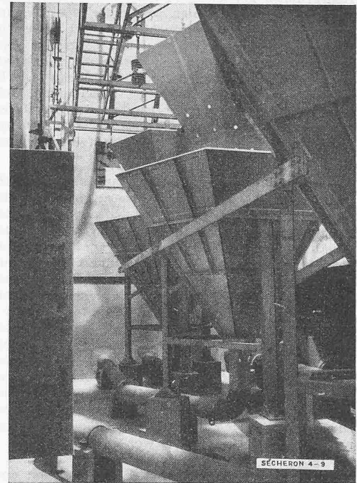
Abb. 4. Trichterförmige feste Boden-Elektroden
