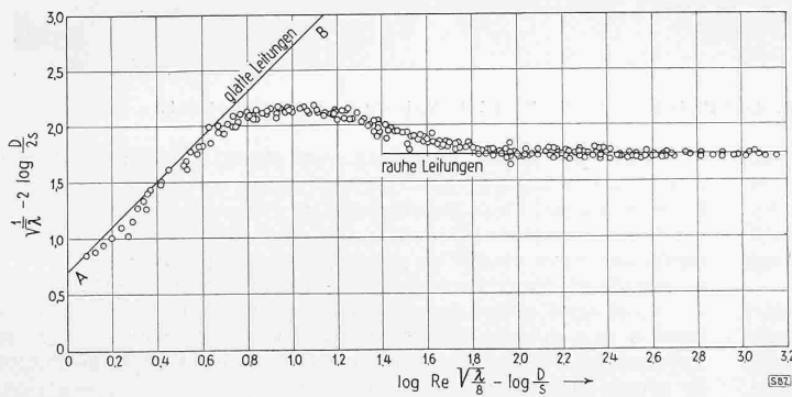
Fig. 6. Courbe de Prandtl-Nikuradse. Variations de λ en fonction du log Re_s*
