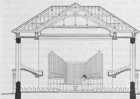
Abb. 4. Querschnitt
