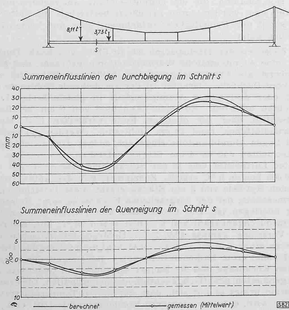
Abb. 3. Vergleich berechneter und gemessener Einflusslinien
