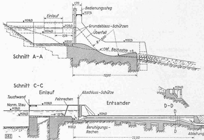
Abb. 4. Schnitte von Wehr und Wasserfassung. — 1:400
