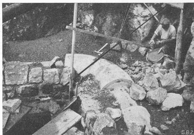
Abb. 6. Winkelpunkt der Hangleitung aus Schleuderbetonrohren
