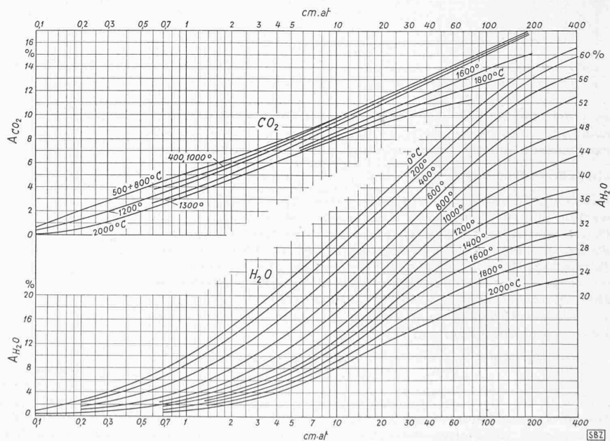
Abb. 2. Gasstrahlung, extrapoliert für p, s > 10 \text{ cm} \cdot \text{at} und \vartheta > 1200^\circ \text{C}
