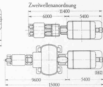
Abb. 11. Abmessungen einer 40/50 000 Heissdampf-turbogruppe alternativ in Ein- und Zweiwellenanordnung. Es sind einer Zweizylinder-Turbine zwei Hochdruck-Zylinder vorgeschaltet, die mit 9000 U/min laufen und ihre Leistungen über ein Getriebe abgeben
