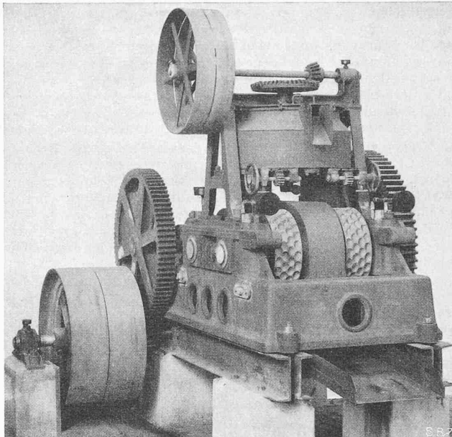
Abb. 14. Brikettpresse von Daverio & Cie., Zürich Die weiche Masse wird aus der über der Presse angebrachten Mischtrommel den Mulden zugeführt und durch den langsamen Drehung der Walzen ausgeübten Druck von bis 50 kg/cm 2 zu eiförmigen Briketts gepresst
