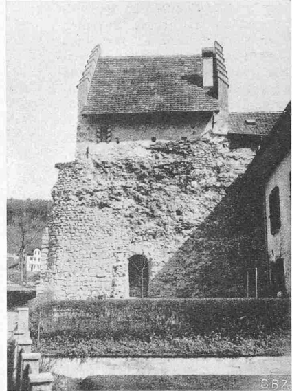
Abb. 5. Römische Mauer der Südfront
