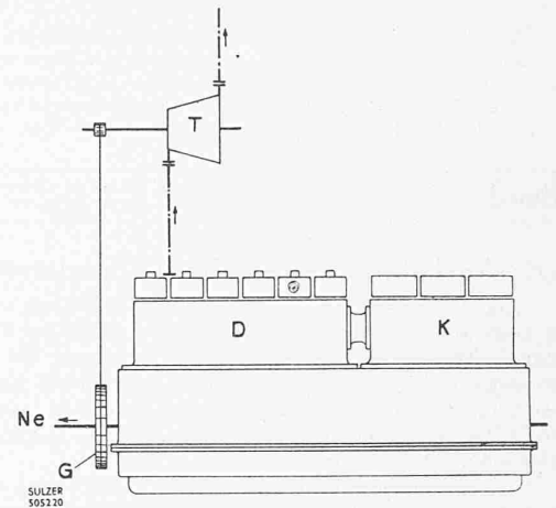
Abb. 5. Schema eines «hochgeladenen» Zweitakt-Dieselmotors mit direkt gekoppeltem Pleuellager. (Dieses Aufladeverfahren ist beim Zweitaktmotor nicht realisierbar, weil die vom Aufladeaggregat gelieferte Spül- und Aufladeluft beim Anlassen und bei kleinen Lasten nicht genügt)
