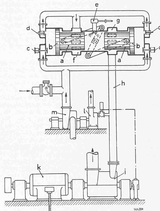
Abb. 7. Schema des «Treibgasverfahrens» mittels Freikolben-Treibgaserzeugers. Die beiden Dieselmotoren a mit den angebauten Kompressor-Kolben b sind durch eine Synchronisierungsvorrichtung derart miteinander verbunden, dass sie sich gegenüber der Totraummitte spiegelbildlich bewegen. Die beiden Dieselmotoren werden durch die Expansion der im schädlichen Raum der Kompressor-Kolben verdichteten Luft zurückgeworfen und kromprimieren dabei die im Dieselmotor enthaltene Luft. Der durch die Düse e eingespritzte Brennstoff wird in der hochverdichteten Luft verbrannt, worauf die beiden Dieselmotoren nach aussen gedrängt werden. Dabei wird die von den Kompressor-Kolben während des vorhergehenden Hubes angesaugte Luft verdichtet. Die geförderte Druckluft dient der Spülung und Aufladung des Dieselmotors. Die als Treibgase bezeichneten Abgase treiben die mit einem Elektro-Generator k gekuppelte Abgasturbine i an. Die Hilfsturbine l, die ebenfalls an die Treibgasleitung angeschlossen ist, treibt den Vorverdichter m an, der die von den Kompressoren angesaugte Luft vorverdichtet und die Kompressoren dadurch auflädt.
