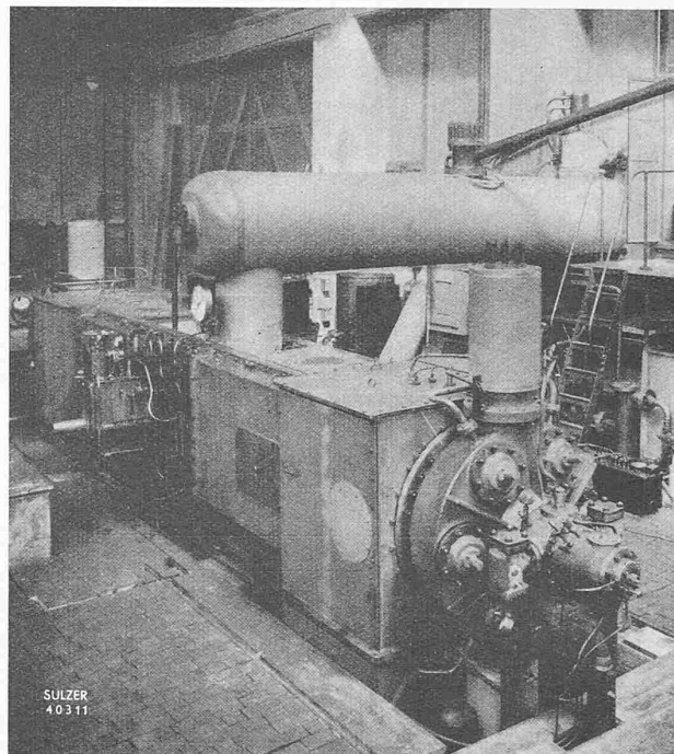
Abb. 8. Versuchs-Freikolben-Treibgaszerzeuger auf dem Versuchstand von Gebrüder Sulzer in Winterthur
