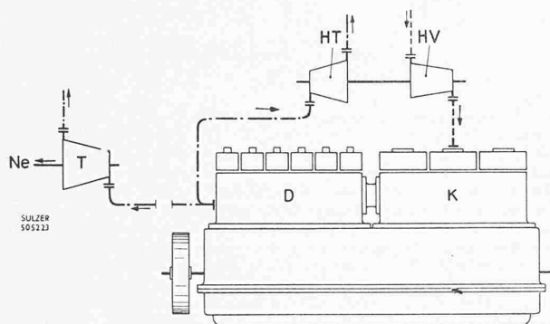
Abb. 9. Schema des «Treibgasverfahrens» mit Vorverdichtung für Aufladepertes von 6 bis 10 ata. Da die erforderliche Verdichterleistung die Dieselmotorleistung übertrifft, wird ein Teil der Treibgasenergie dazu verwendet, die fehlende Verdichterleistung zu decken.
