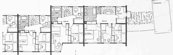
GRUNDRISS OBERGESCHOSS M. 1:400
