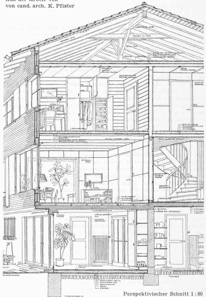
Perspektivischer Schnitt 1:80
