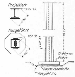
Abb. 23. Querschnittänderung Säule 28 von rechteckig auf rund. — 1 : 80
