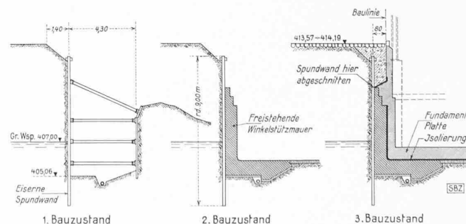
Abb. 19. Bauvorgang beim Betonieren der Umfassungswände. — 1 : 300
