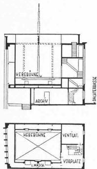
Abb. 11. Reklamenturm Masstab 1 : 600
