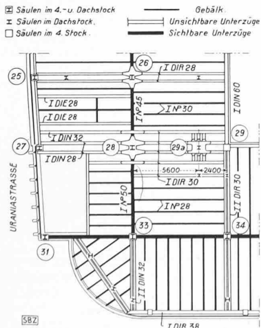
Abfangung der Säule 29a in der Decke über dem 1. Stock
