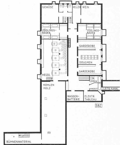
Abb. 11. Kellergrundriss 1 : 500
