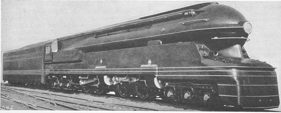
Abb. 1. American Railroads Lokomotive 3BB3, 6500 PS, für 160 km/h bei 1100 t Anhängewicht
