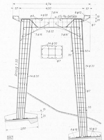
Abb. 7. Brückenjoch 1:120
