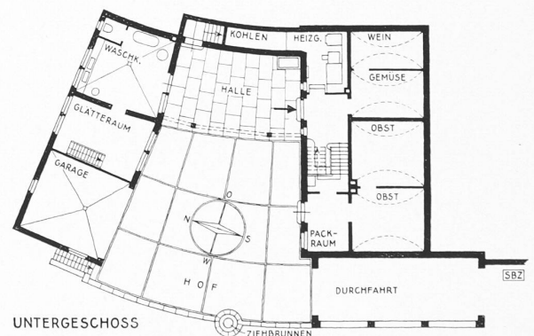
Abb. 18. Schnitte (vergl. Abb. 15). — 1: 400. — Abb. 17 (unten). Untergeschoss
