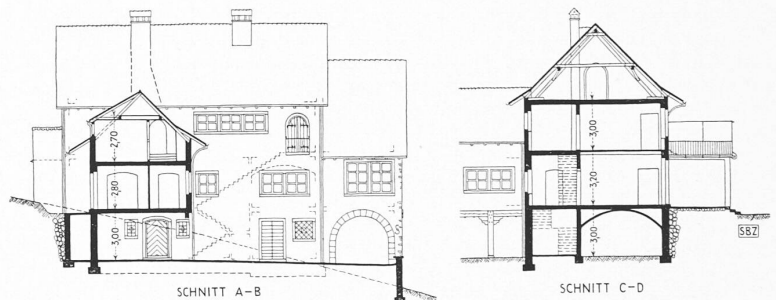
Abb. 18. Schnitte (vergl. Abb. 15). — 1: 400. — Abb. 17 (unten). Untergeschoss
