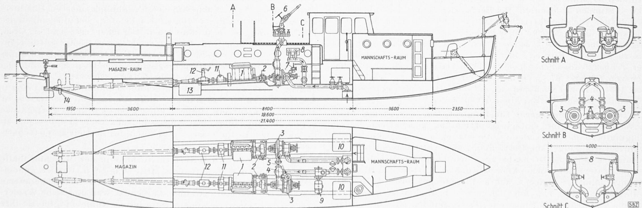
Abb. 2. M. S. «Sankt Florian», Grundriss u. Schnitte 1:150. — Legende: 1 Dieselmotoren, 2 Brennkupplungen, 3 Feuerlöschpumpen, 4 Rückschlagklappen, 5 Umstellschieber für Seriebetrieb, 6 Wasserkanone, 7 Vakuumpumpe, 8 Bergungs-Anschlüsse, 9 Hilfsaggregat 8 PS, 110 V Gleichstrom, 10 Brennstoffbehälter zu je 350 l, 11 Reduktionsgetriebe, 12 Steuerventile, 13 Steuerölbehälter, 14 Verstellpropeller \varnothing 800
