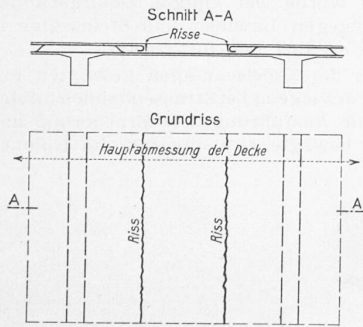
Abb. 15a. Plattenbalkendecke
