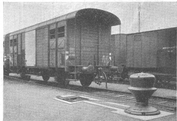
Rangierspilanlage SBB Werkstätte Zürich-Altstetten
