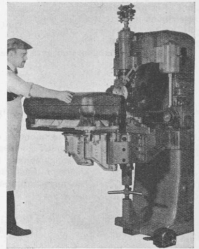
Abb. 7. Nahtschweissmaschine
