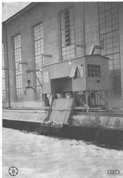
Rechenreinigungsmaschine Klingnau
