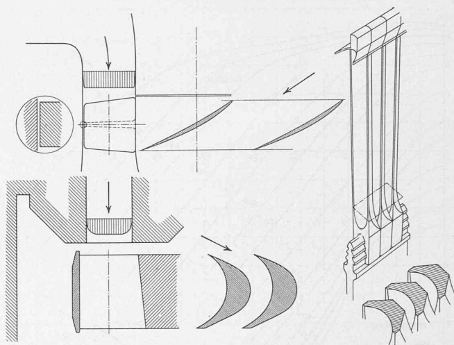
Abb. 17. Vergleich der Ausführungseinheit von Kaplan-Turbinen (oben) und Dampfturbinen (unten). Auch bei sehr guten Konstruktionen (rechts) gibt es Schnitte, wo die Dampfströmung sehr ungünstig sein muss
