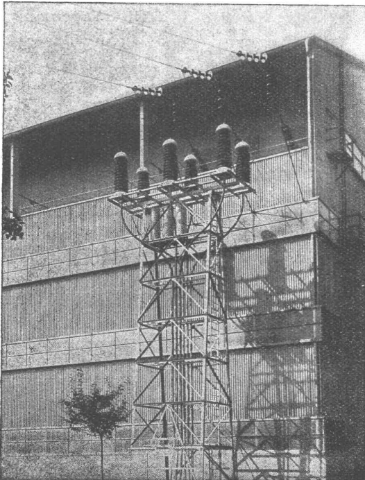
150 kV-Ölkabelanlage im Unterwerk Töss der Nordostschweizerischen Kraftwerke
