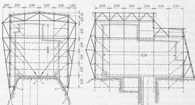
Abb. 9. Konstruktions-System der Schutzhütte. — 1:350
