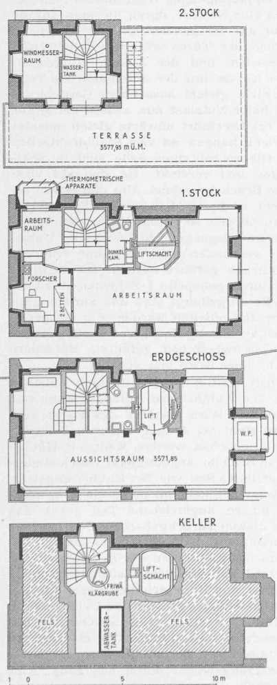
Abb. 16. Grundrisse. Masstab 1:250
