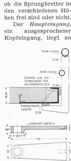
Abb. 18 (oben). Detail 1:10 des Treppen-Geländers, darunter: Betonelement der Treppe, 1:50
