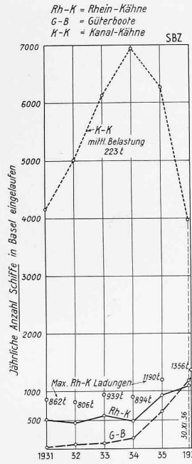
Abb. 5. Anzahl Schiffe 1931/36.
