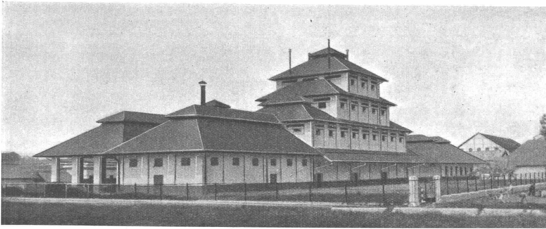
Brauereianlage in Soerabaja, Java. Gebäulichkeiten: Schwebende Pfahlfundierung mit 500 Eisenbetonpfählen, Eisenbetonrost, Skelettbau in Eisenbeton, eiserne Dächer mit Ziegelabdeckung, Ausmauerung mit Backsteinen. Text dazu siehe Seite 30.
