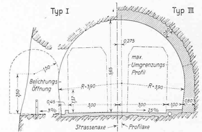
Abb. 7. Galerie-Normalprofile 1 : 200
