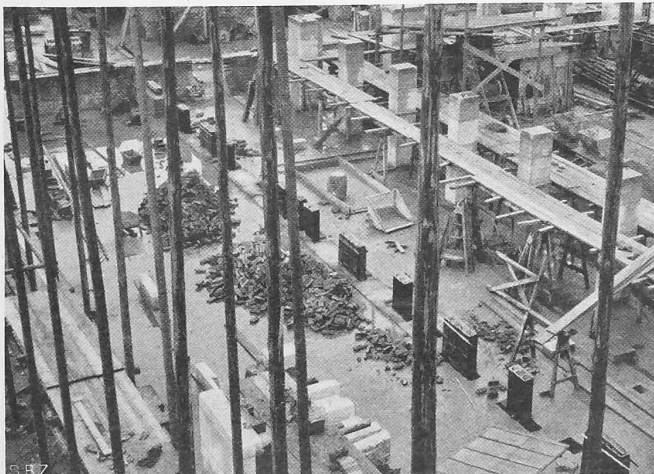
Abb. 9. Baubild mit den aufsteigenden Lüftungskanälen.
