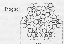
Abb. 11. Seilprofile.
