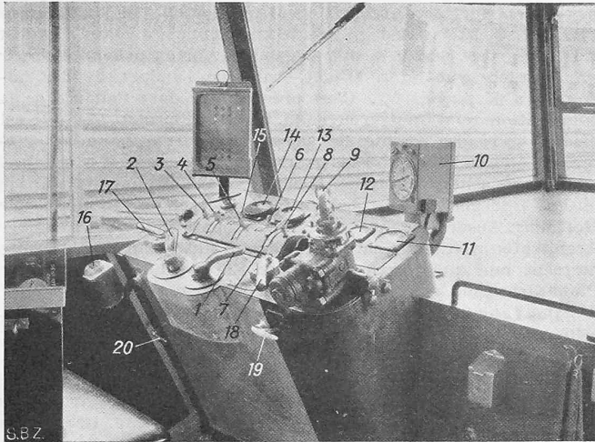
Abb. 5. Führerpult. — Legende: 1 Stufengetriebehebel, 2 Motorregulierung, 3 Abstellschalter, 4 Anlassschalter, 5 Kompressorschalter, 6 Steuerstromschalter, 7 Wendegtriebeschalter, 8 Entriegelungsschlüssel, 9 Führerbremventil, 10 Geschwindigkeitsmesser, 11 und 12 Bremsluft-Manometer, 13 Kühlwasserthermometer, 14 Motor-Tachometer, 15 Fernschalter für Luftheizung, 16 Wachsamkeitstaste, 17 Betätigungshebel zu Türen links, 18 desgl. rechts, 19 Pfeifenzug, 20 Hahn zu Fensterwischer.
