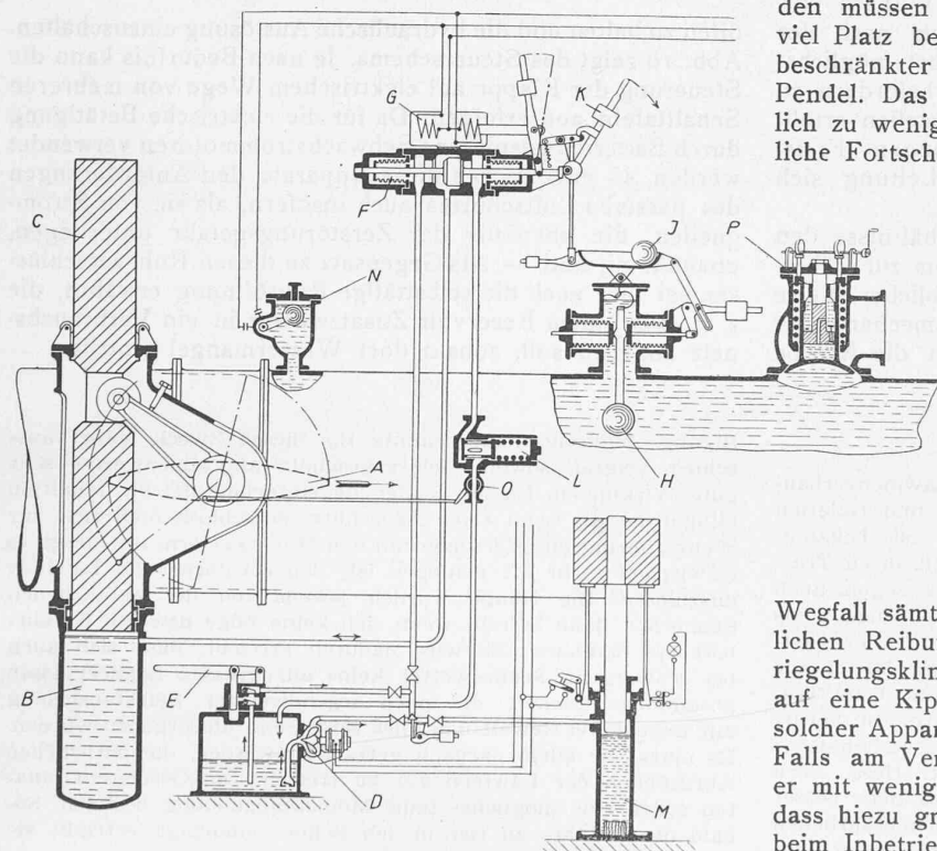
Abb. 7a. Steuerschema eines selbsttätigen Rohrabschlusses mit hydraulischem Oeffnungszylinder und Fernsteuerung. A Drosselklappe, B Servomotor-Oeffnungszylinder, C Schliessgewicht, D Motorpumpe, E Handpumpe, F Steuerventil, G Steuermagnet, H Hydr. Auslösung, J Verstärker, K Fallgewicht, L Druckreduzierventil, M Akkumulator, N Schwimmertopf, O Drosselapparat, P Autom. Lufteinlassventil.
