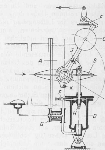
Abb. 6a. Automat. Rohrabschluss mit Schliessgewicht neuer Bauart.
