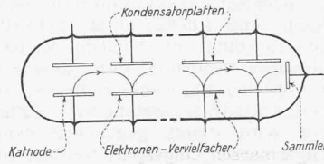
Abb. 5. Elektronenbahn in der magnetischen Elektronen-Vervielfacher-Photozelle.
