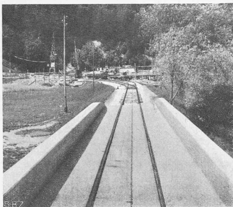
Abb. 17. Einbetoniertes Normalspurgeleise.
