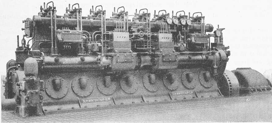
Abb. 7. 330 PS-Schiffs-Dieselmotor „SLM-Winterthur“ mit angebautem Wendegetriebe MWP, zwei ganze Maschinen-Ausrüstungen für Boote gemäss Abb. 6 geliefert von der „SLM-Winterthur“.
