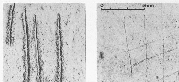
Abb. 2. Oberflächen-Struktur von PZ 300 plastisch, links ohne und rechts mit Plastimentzusatz. Das Vorhandensein bzw. Fehlen der Schlammschicht ist durch Ritzen der Oberfläche veranschaulicht.
