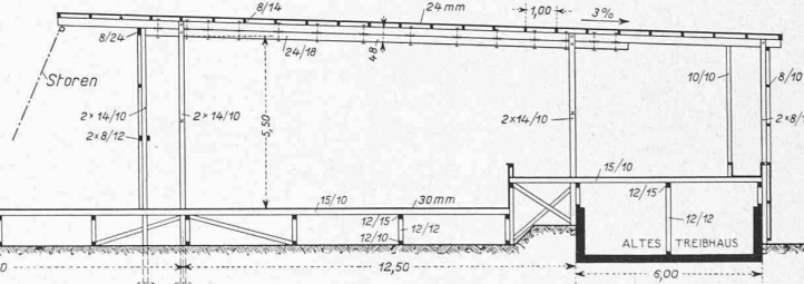
Abb. 10 und 11. Restaurant; hölzernes Skelett. Ansicht Südwand und Querschnitt (Dreifache Stufung — Terrain, Boden, Estrade — wegen Fernsicht). — 1 : 250.
