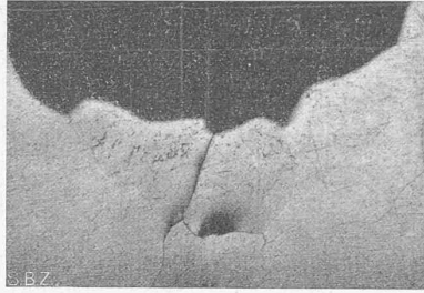
Abb. 26. Mikrophotographie eines korrodierten Messings mit interkristallinen Rissen. 50 fach.
