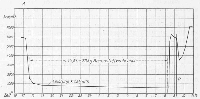
Abb. 4. Regulierversuch (Nachtbrand) an einem Kessel von 33,5 m 2 Heizfläche. A nach 10 Stunden Brenndauer ohne Entschlacken, Teilfüllung aufgegeben und Luftdrosselklappen geschlossen. B Entschlacken und Aufgabe einer Teilfüllung.
