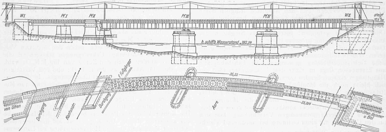
Abb. 1. Aarebrücke der „Gäubahn“ bei Olten. Berechnet, konstruiert und ausgeführt von der A.-G. Th. Bell & Cie., Kriens (Obering. F. Ackermann). — Rd. 1 : 800.
