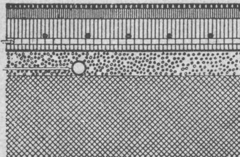
Patentierte „Isolaphon“-Unterlagsboden
