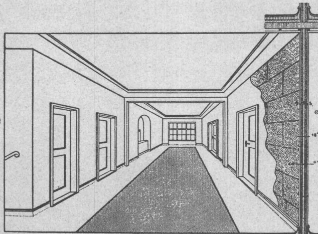
Patentierte „Isolaphon“-Leichtwände
