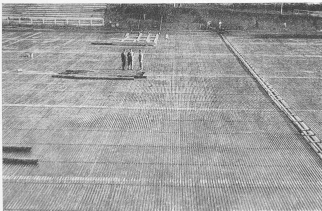
Abb. 3. Teilansicht des Rohrfeldes der Dolder-Eisbahn.
