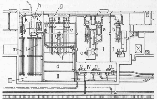
Abb. 5. Querschnitt und Grundriss der Maschinenanlage, 1 : 300.
