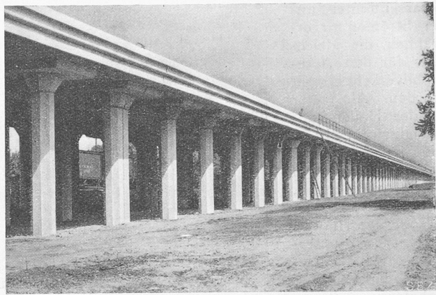
Abb. 54 und 55. Viergeleisiger Viadukt in amerikanischer Pilzdeckenform für die Bahnhof-Erweiterung in Columbus (Ohio) der Pennsylvania R. R.
