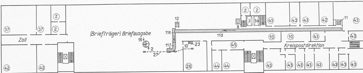
Abb. 22. Schematischer Grundriss vom 2. Obergeschoss des Hauptgebäudes. — Masstab 1 : 700.
