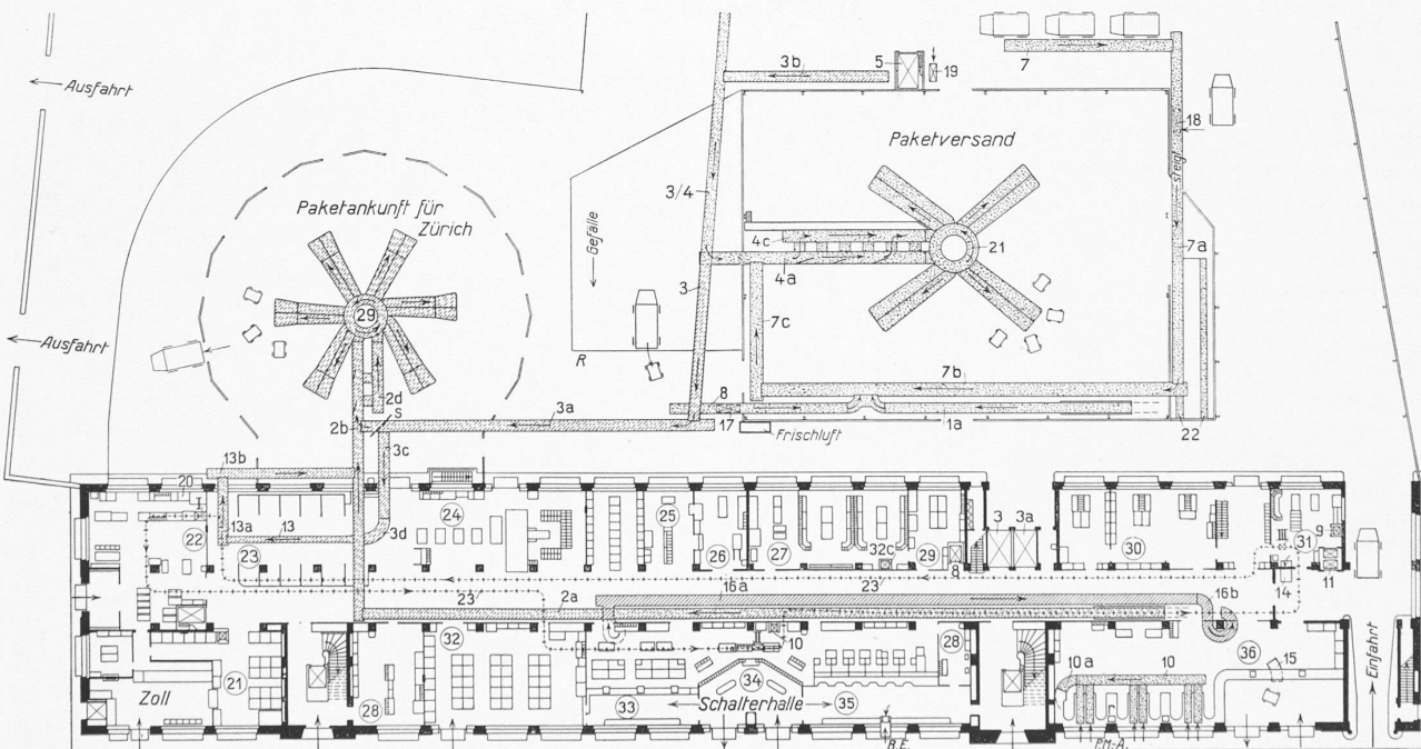
Abb. 20. Grundriss vom Erdgeschoss des Hauptgebäudes und der Anbauten für Paketausgabe und Paketversand. — Masstab 1 : 700.
