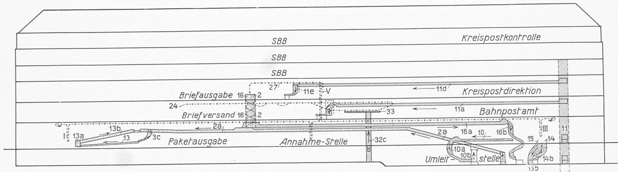
Abb. 23. Schematischer Längsschnitt durch das Hauptgebäude der neuen Sihpost in Zürich. — Masstab 1 : 700.
