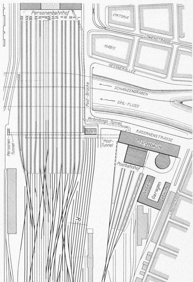
Abb. 1. Der Postbahnhof neben dem Personenbahnhof Zürich. — 1 : 4000.
