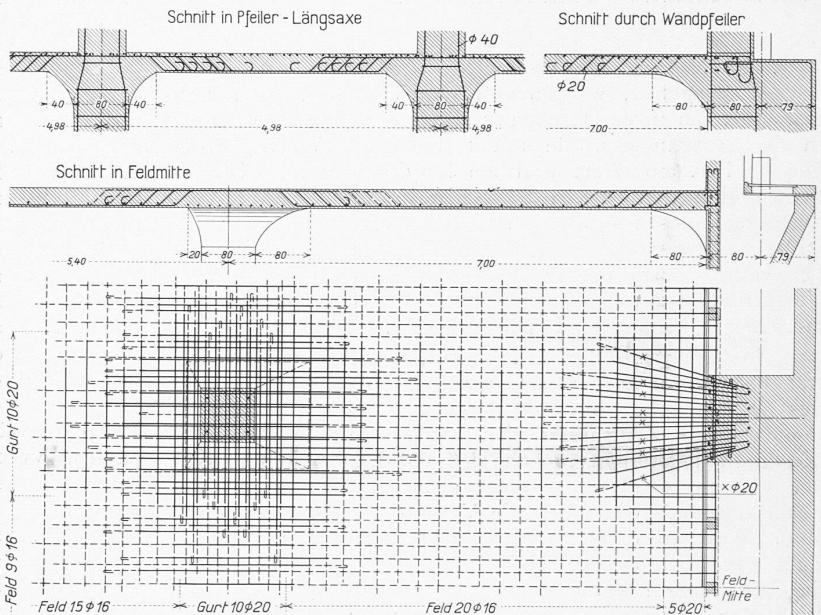
Abb. 45. Pilzdecke im Anbau-Untergeschoss (Sackstückversand).
