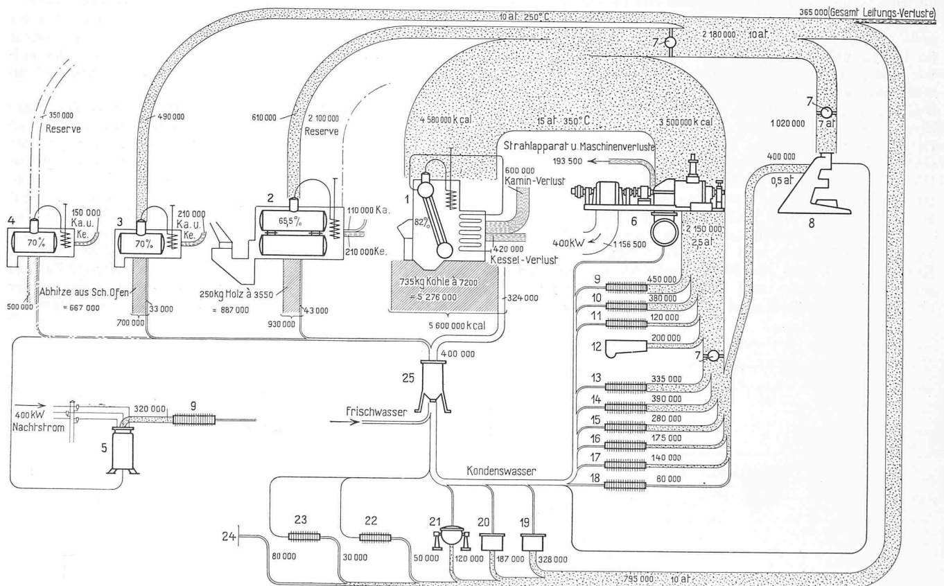
Abb. 6. Wärmebilanz des Heizkraftwerkes der Schweizer Industrie-Gesellschaft Neuhausen bei 0° C Aussentemperatur.
