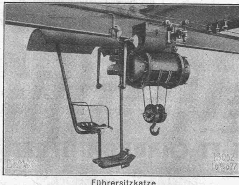
Führersitzkatze
