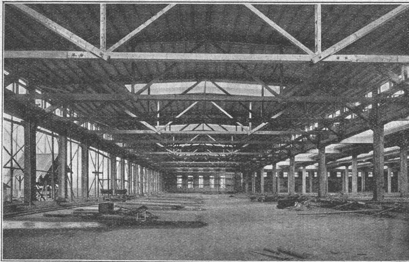
Lokomotivremise der S.B.B. in Zürich Spannweite 24,40 m
